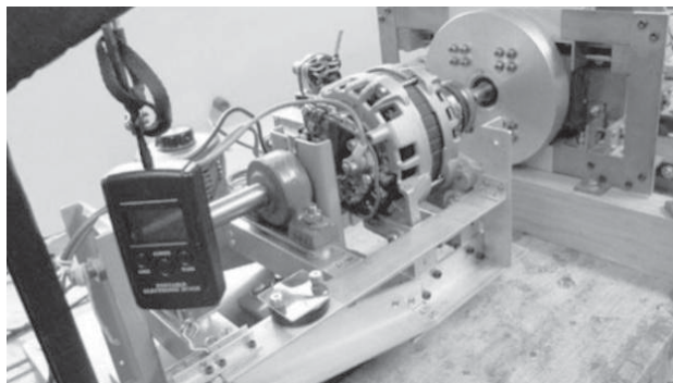
Especialistas del INTI realizaron ensayos sobre el nuevo motor y la fuente realimentadora.(Inti/InfoGEI)
